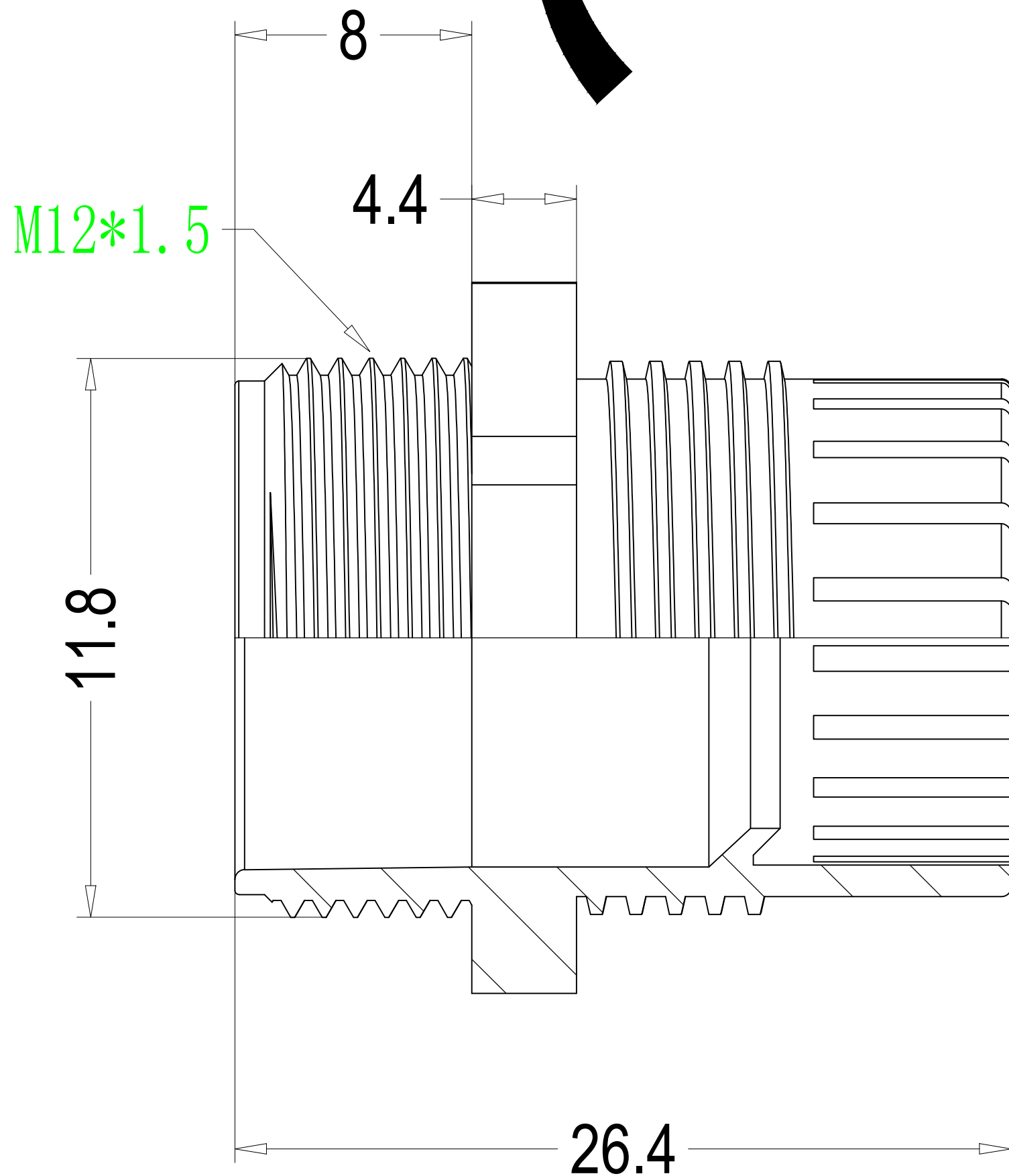
本体 Body
