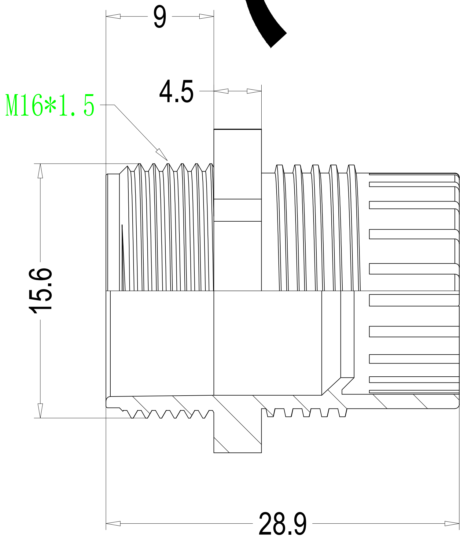
本体 Body
