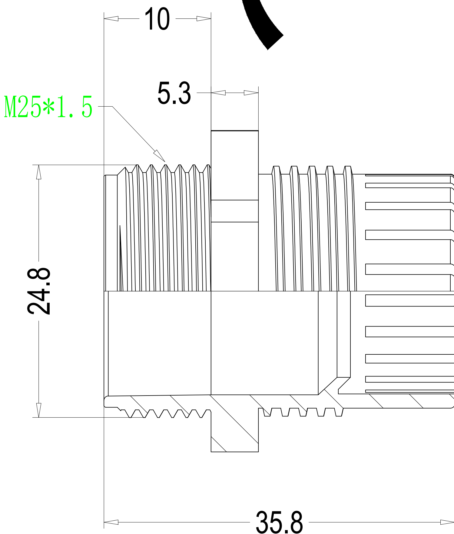
本体 Body
