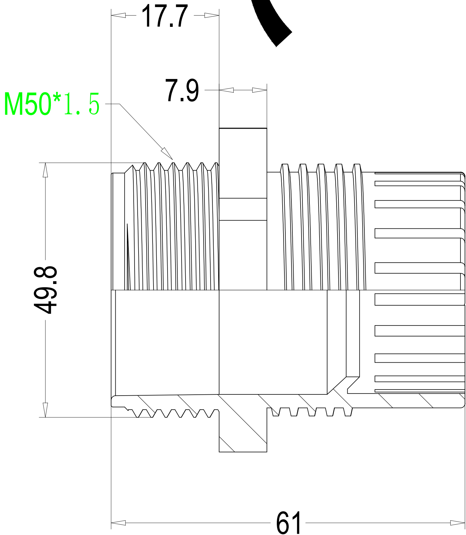
本体 Body
