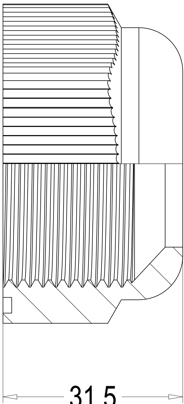
迫紧头 SealingNut
