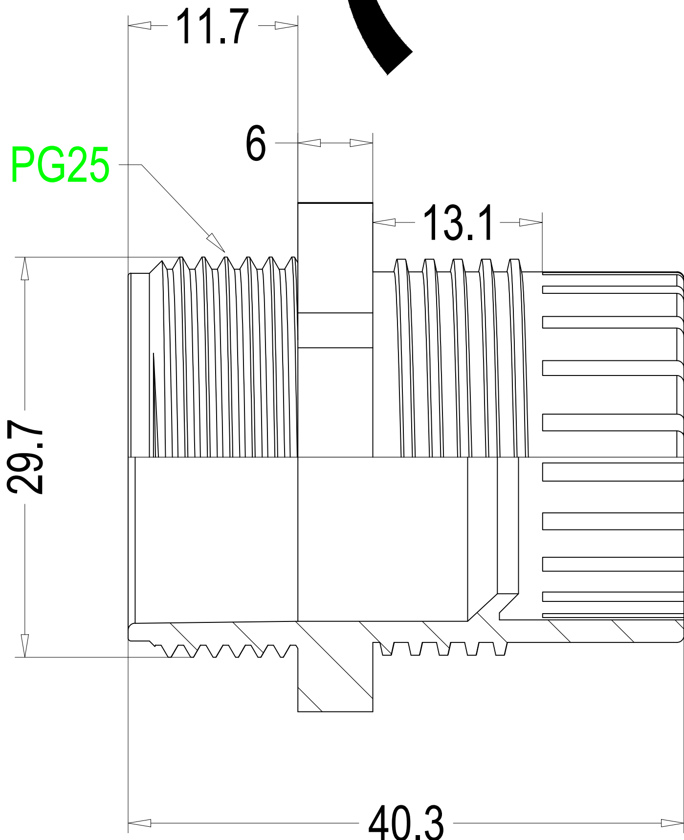
本体 Body C
