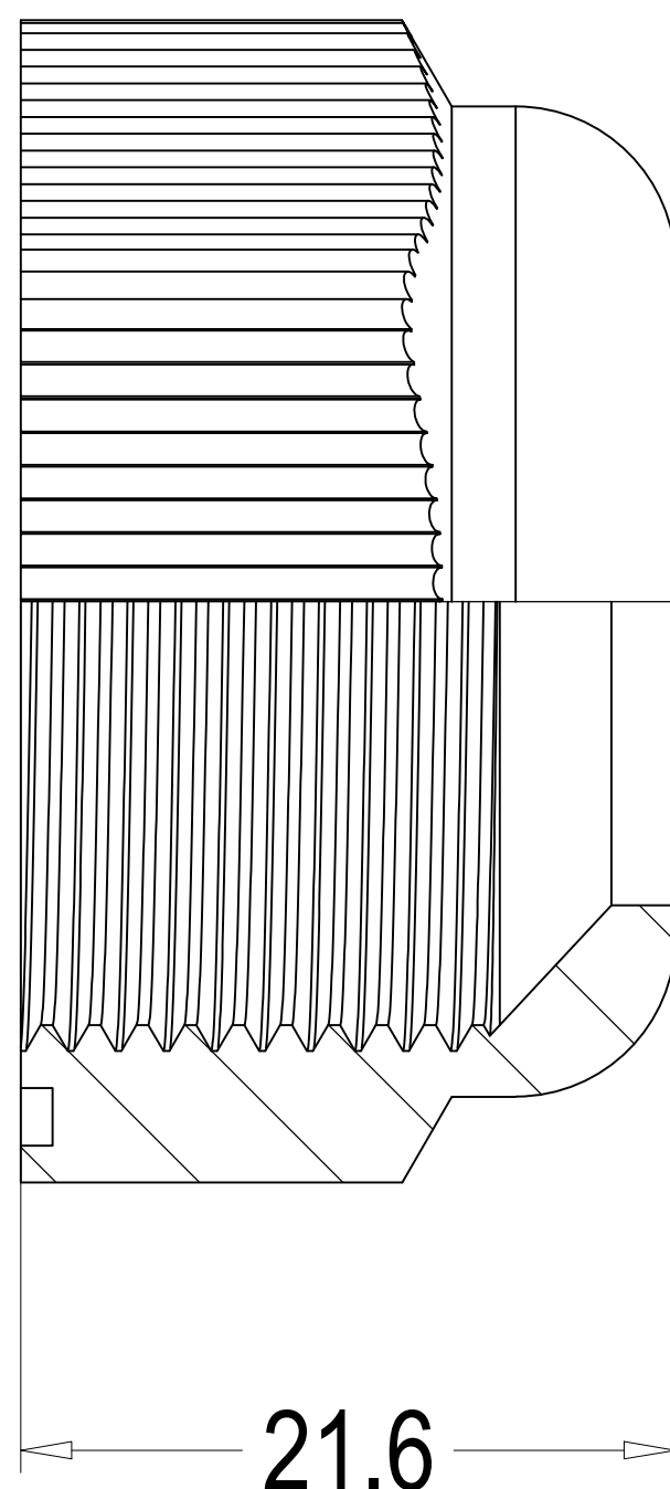
迫紧头 SealingNut F
