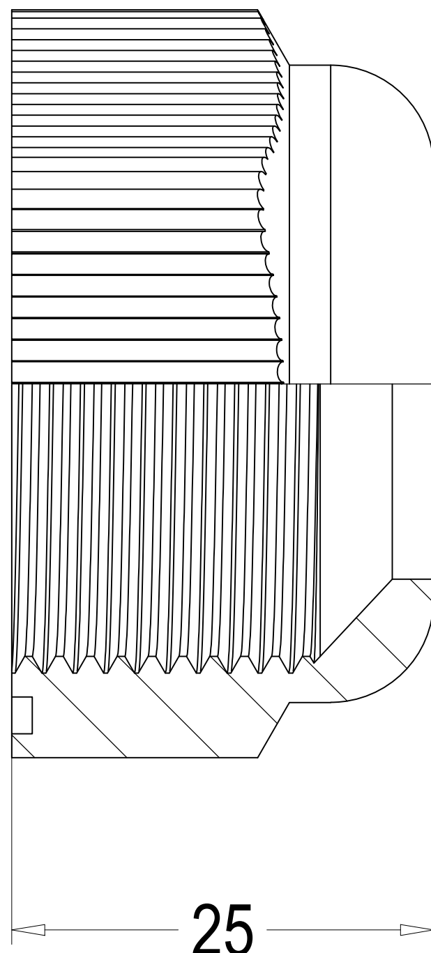
迫紧头 SealingNut
