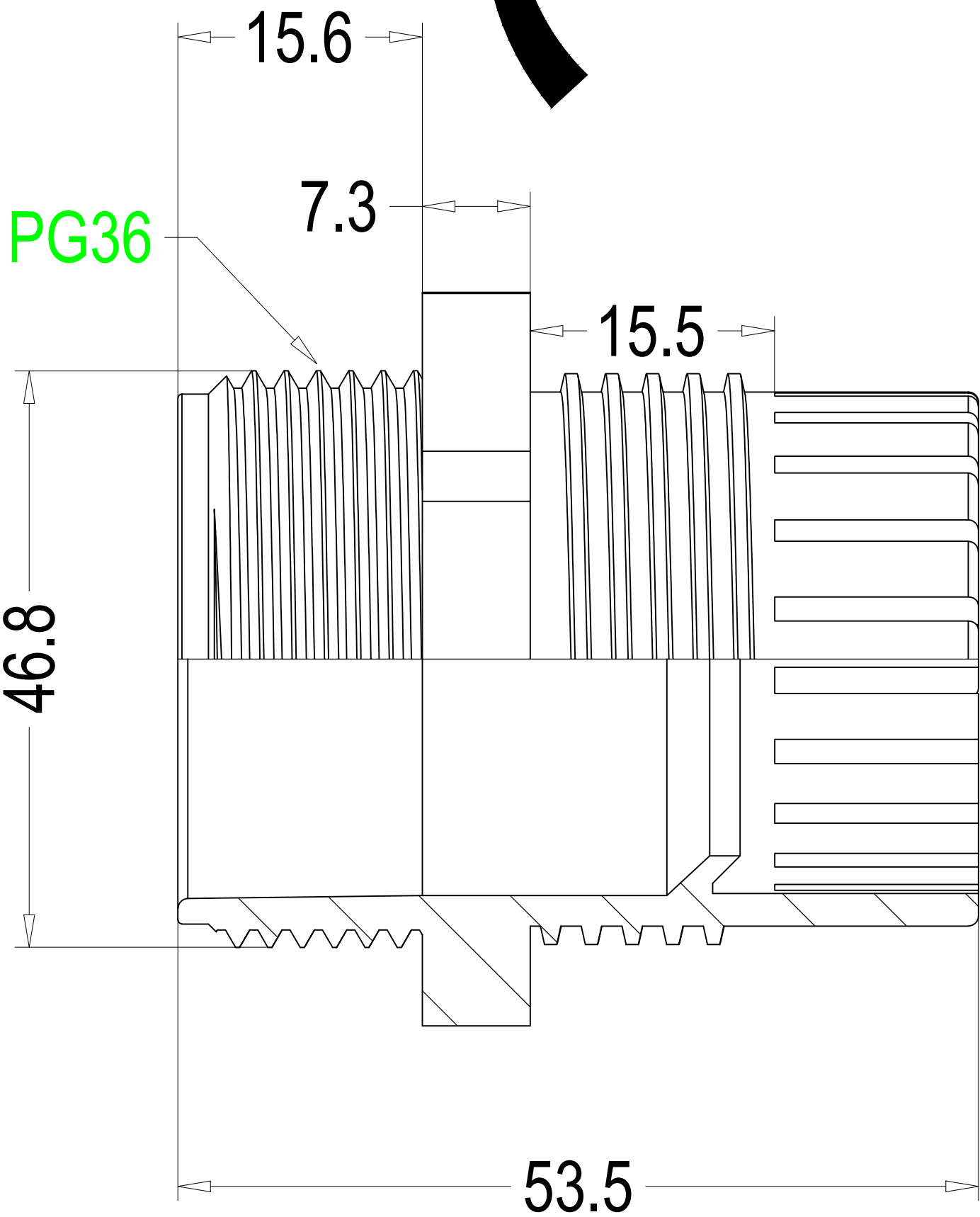
本体 Body C
